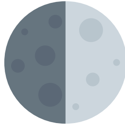
PRIMO QUARTO
