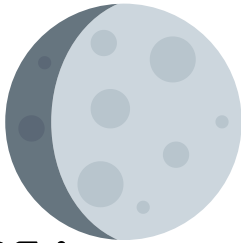
GIBBOSA CRESCENTE
