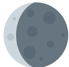
LUNA CALANTE
