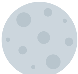
LUNA PIENA
