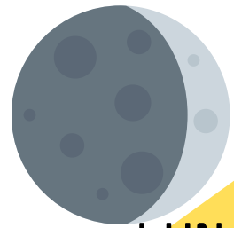
LUNA CRESCENTE
