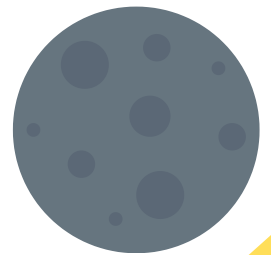
LUNA NUOVA
