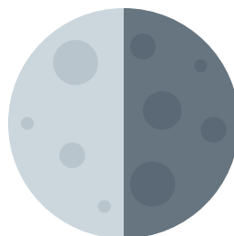
ULTIMO QUARTO
